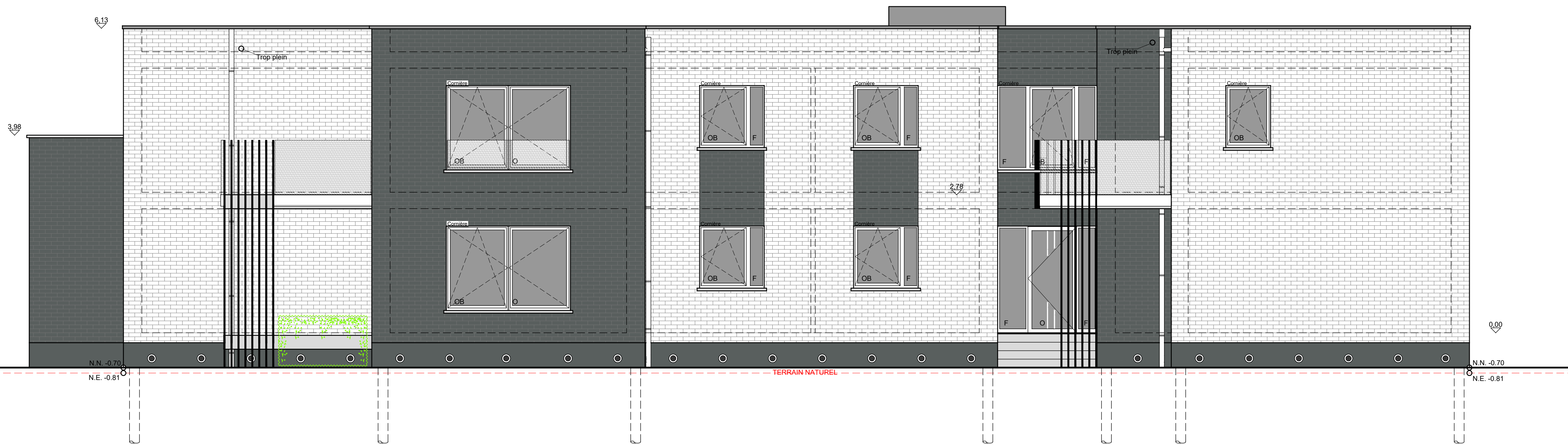
VUES EN ELEVATION (SUD-EST) - 1/200
