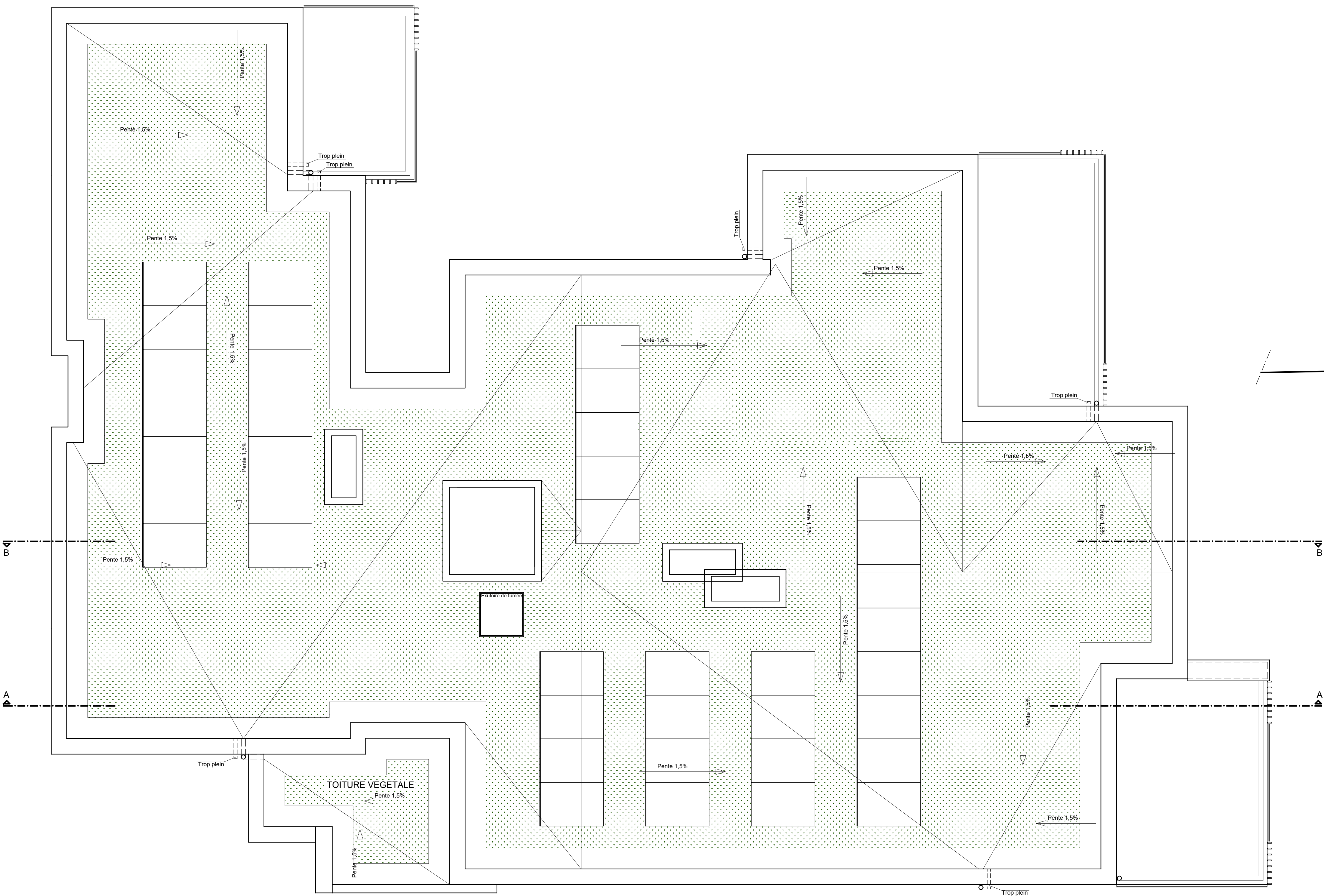
PLAN DES TOITURES - 1/50
