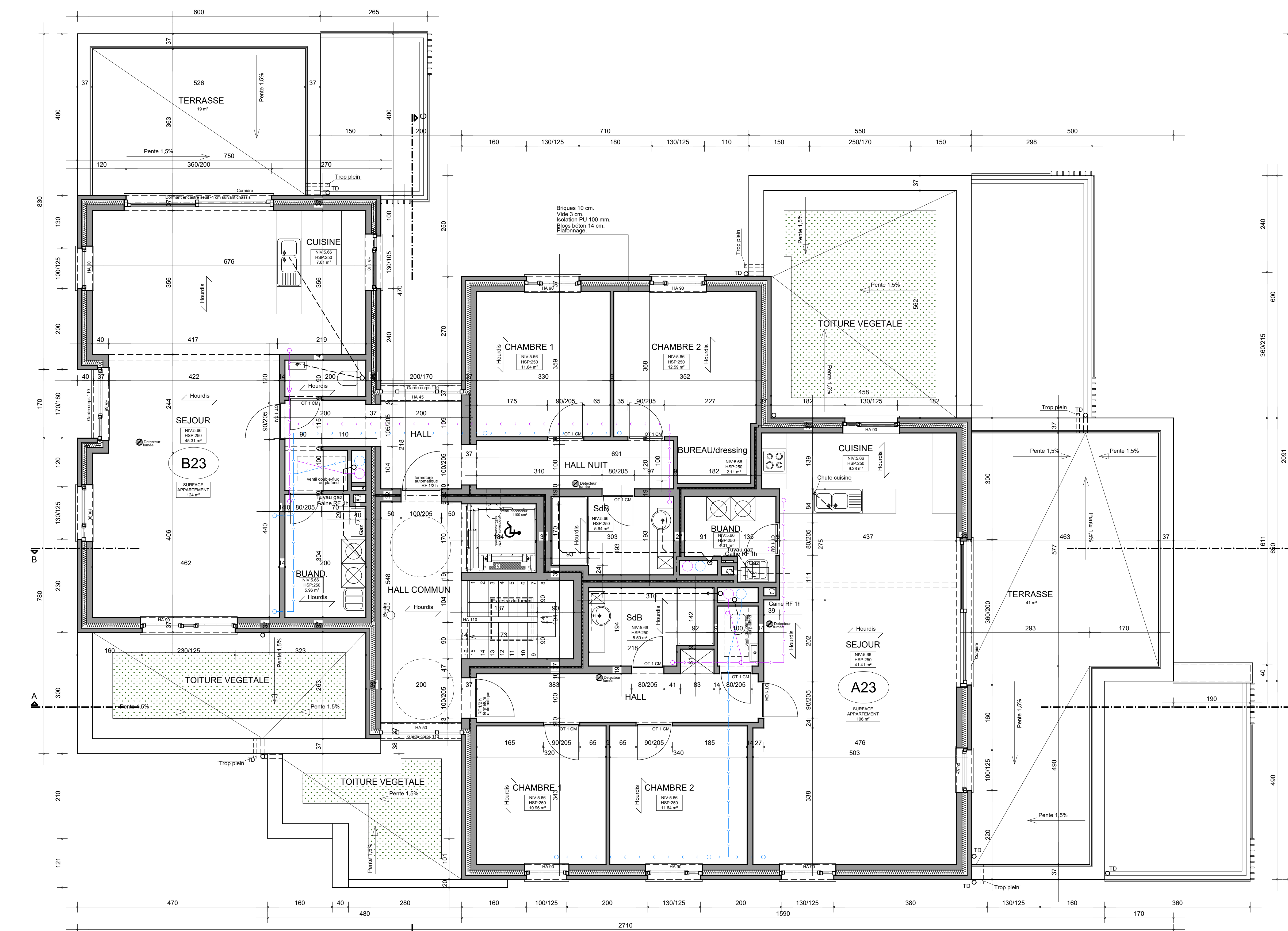
PLAN DU DEUXIEME ETAGE - 1/50
