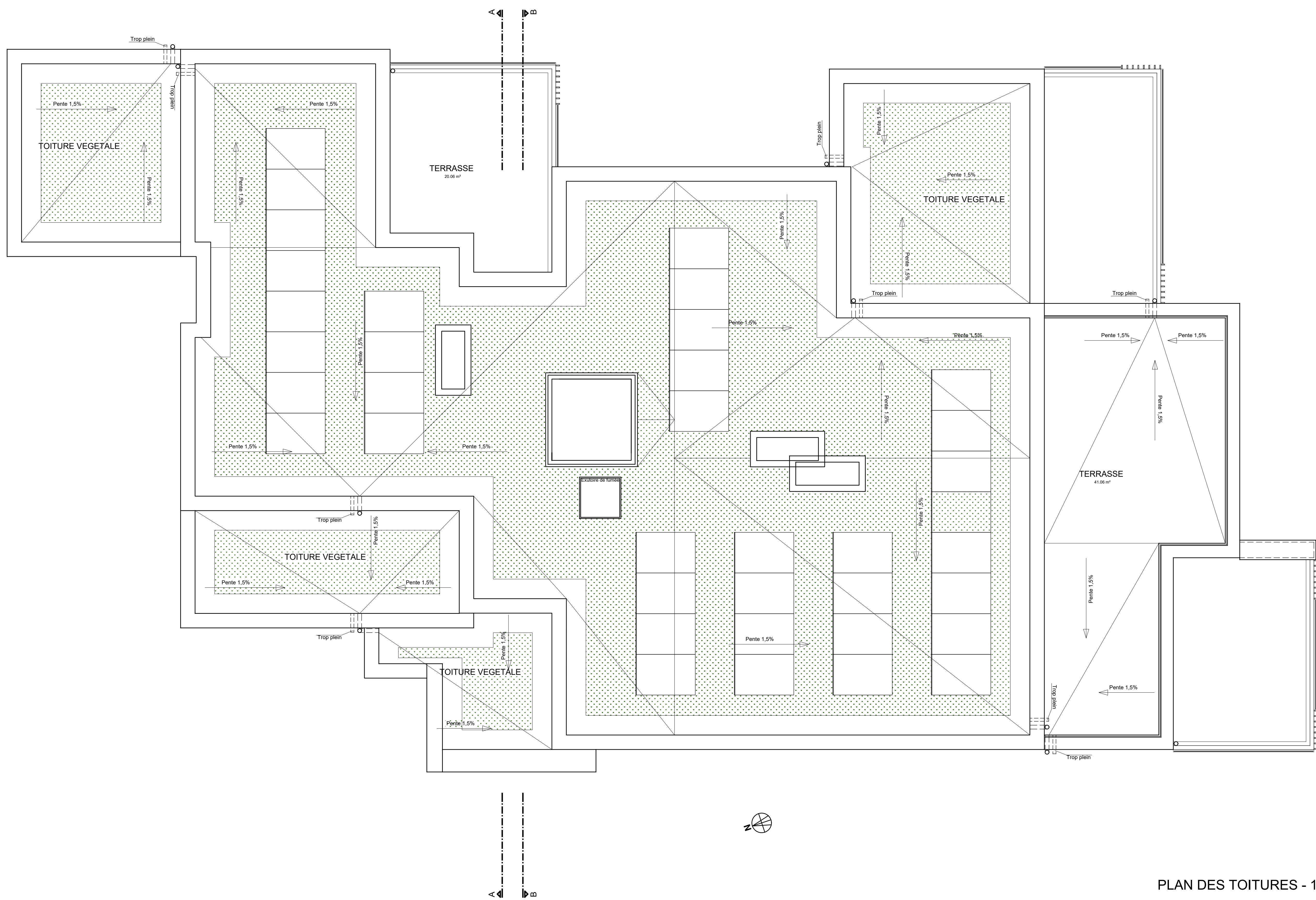
PLAN DES TOITURES - 1/50
