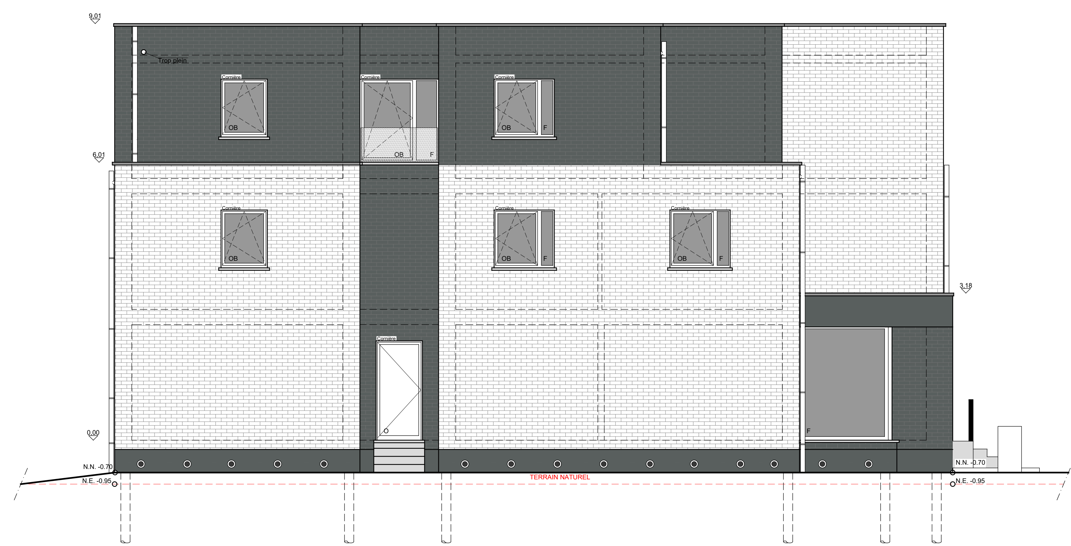
VUES EN ELEVATION (NORD-EST) - 1/200
